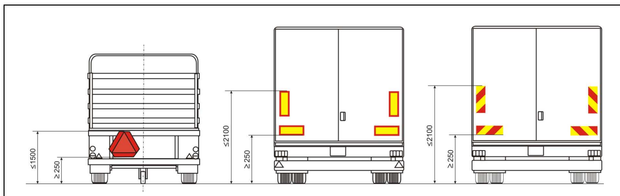
Obr. 1.: Dosiaľ povinné reflexné označenia vozidiel v SR. Vľavo označenie pomalého vozidla podľa predpisu EHK č. 69 (v SR do 40 \text{ km.h}^{-1} ), uprostred označenie dlhého prípojného vozidla podľa predpisu EHK č. 70 (v SR vozidlá kategórií O_1 až O_3 dlhšie než 8 m vrátane oja a všetky vozidlá kategórie O_4 ) a vpravo označenie ťažkého nákladného motorového vozidla podľa predpisu EHK č. 70 (v SR nad 7,5 t).
